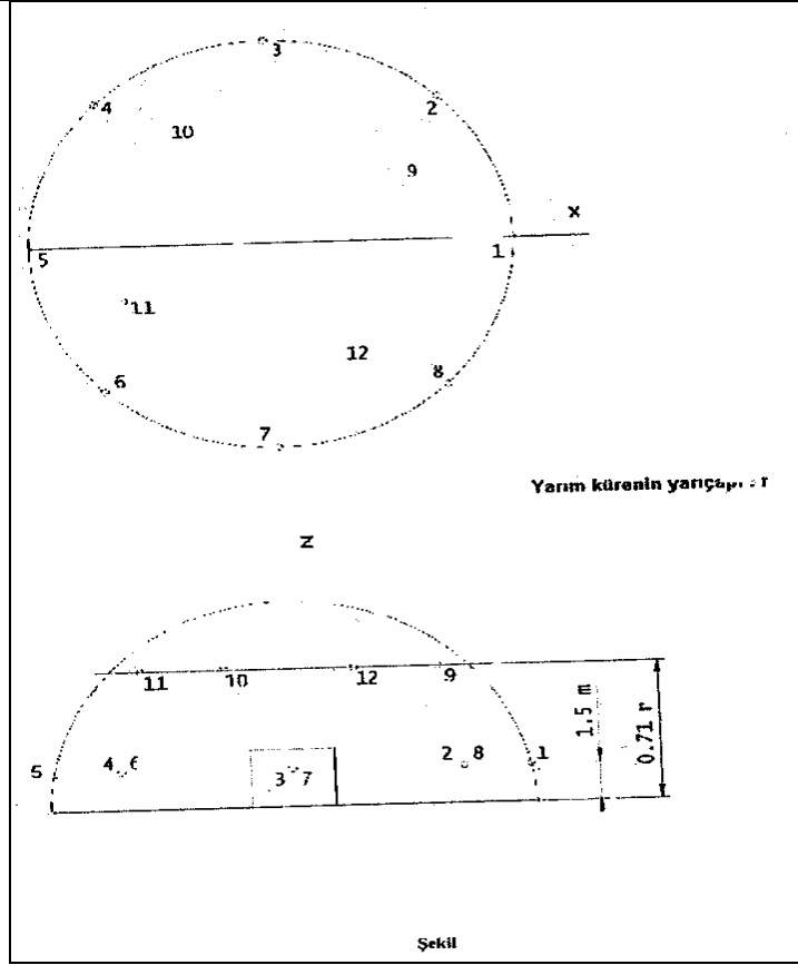
Yarım küre üzerindeki ilave mikrofon dizilişi (12 mikrofonun konumları)
